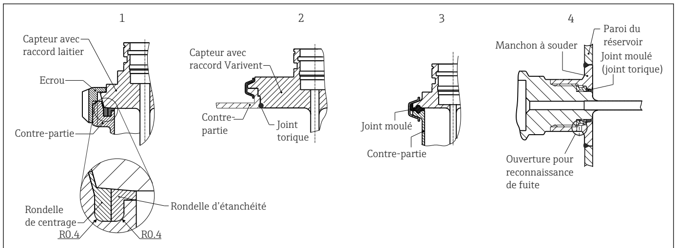
5 Instructions de montage détaillées dans le cas d'une installation hygiénique
