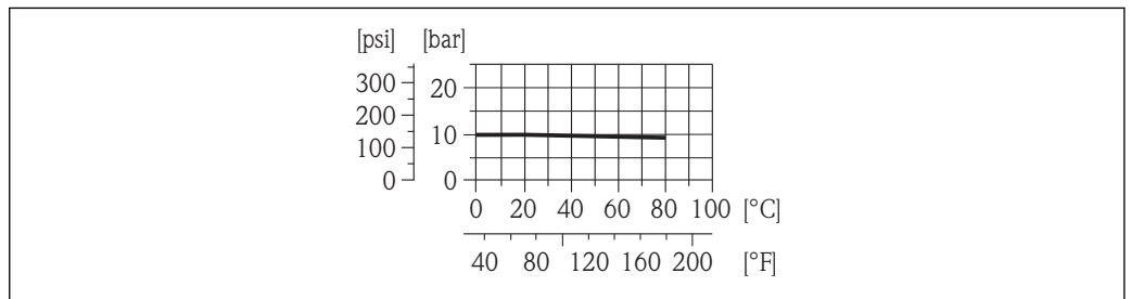
14 Avec bride tournante Class 150, matériaux 1.4404 (316L) et A105 (DN 50 à 200 / 2 à 8")
