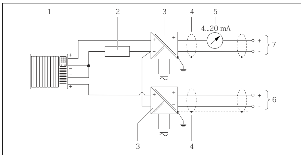
■ 11 Exemple de raccordement pour entrée HART avec "moins" commun
