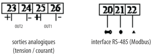
Fig.3. Mode de connexion des signaux de sortie en fonction du code d'exécution.
