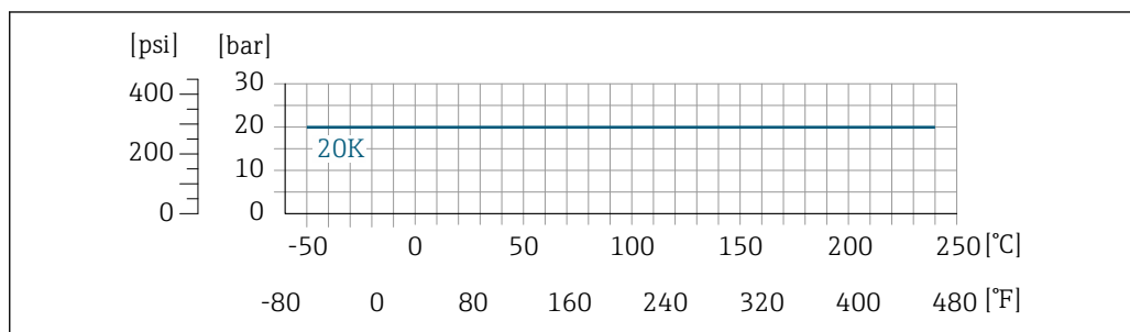
31 Avec matériau de bride 1.4301 (F304) ; pièces en contact avec le produit Alloy C22
