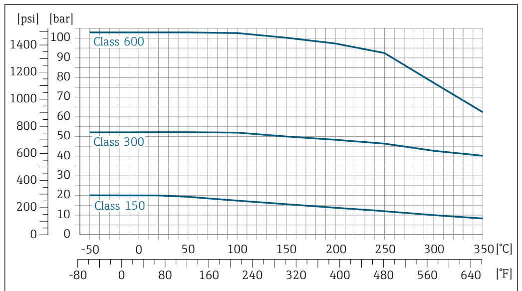
26 Avec matériau de bride Alloy C22
