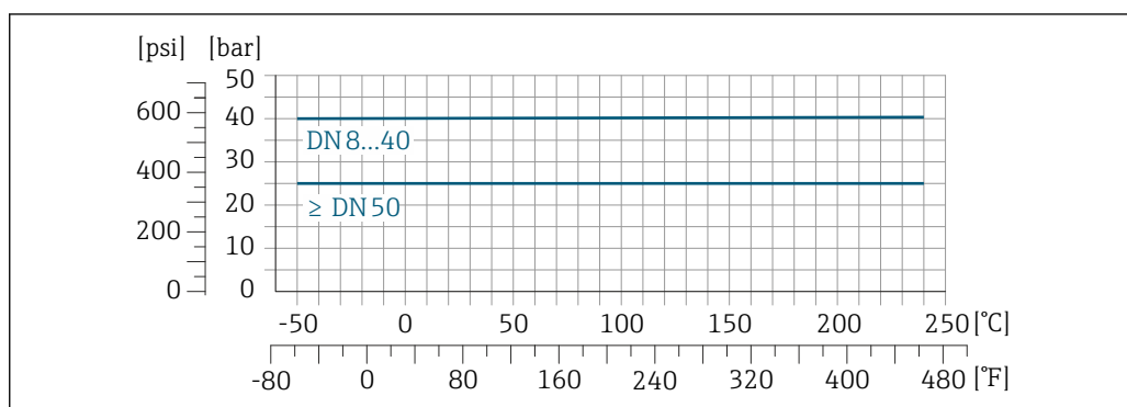
32 Avec matériau de raccord 1.4404 (316/316L)
