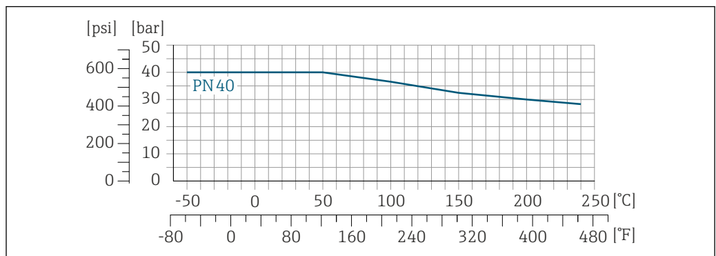
29 Avec matériau de bride 1.4301 (F304) ; pièces en contact avec le produit Alloy C22
