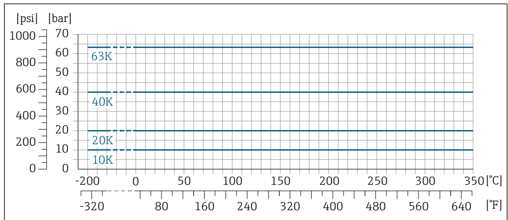
27 Avec matériau de bride 1.4404 (F316/F316L), Alloy C22
