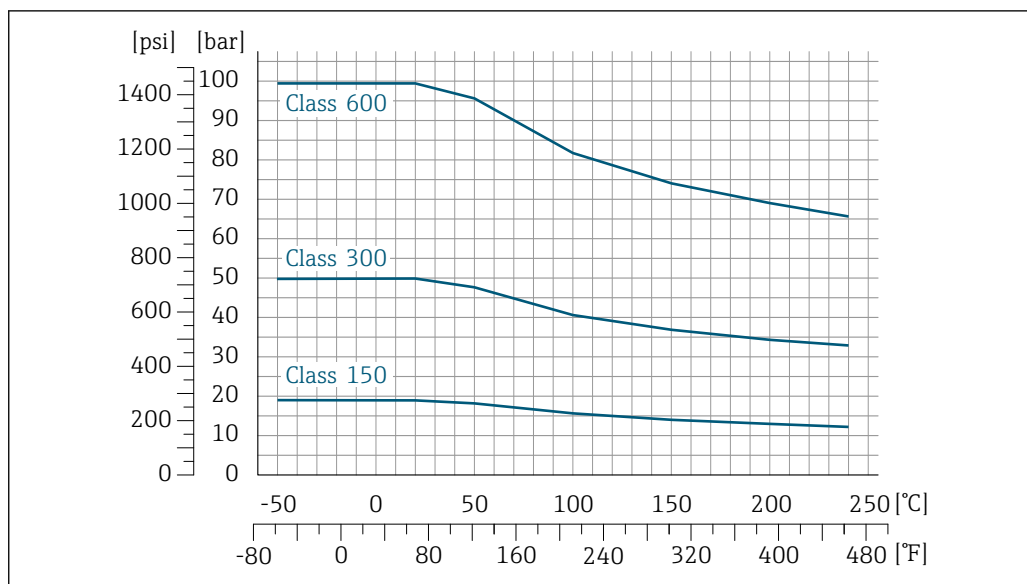
30 Avec matériau de bride 1.4301 (F304) ; pièces en contact avec le produit Alloy C22
