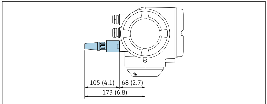
44 Unité de mesure mm (in)
