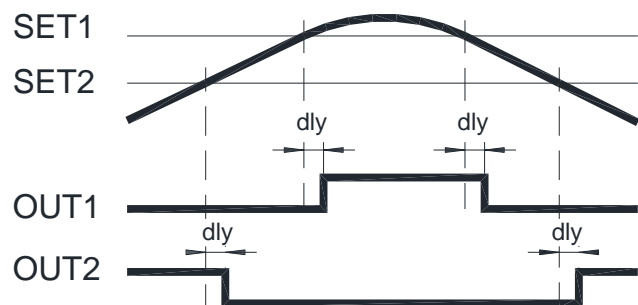
Temporisation en mode HI (SET1-OUT1) et en mode LO (SET2-OUT2).
