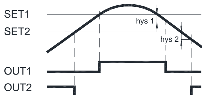
Hystérésis en mode HI (SET1-OUT1-hys 1) et en mode LO (SET2-OUT2-hys-2).
