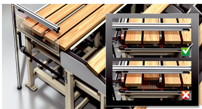
Commutation du transport longitudinal au transport transversal
