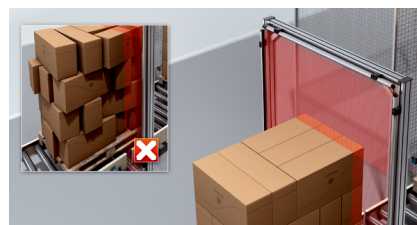
Contrôle de dépassement au niveau des palettes
